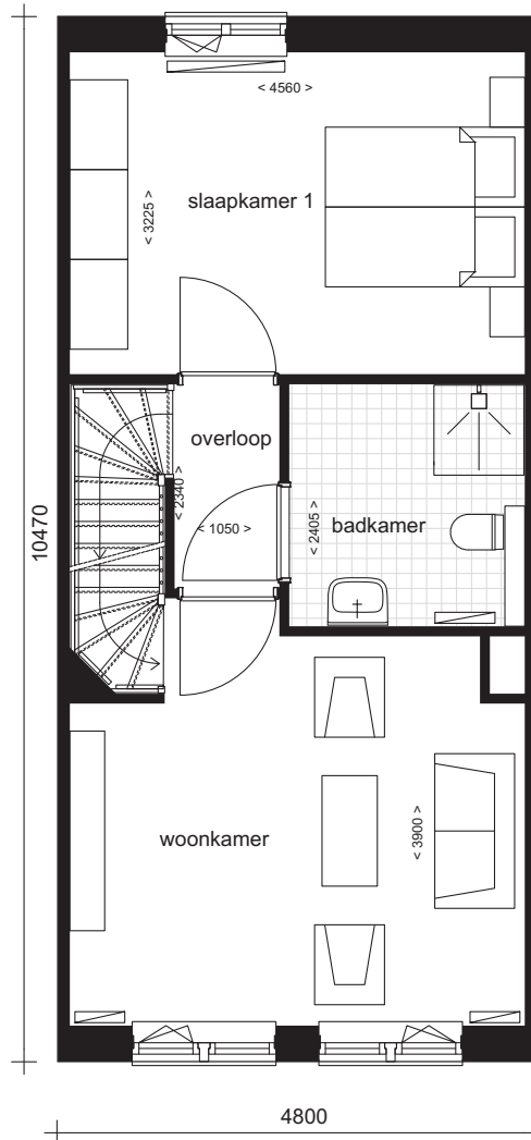
1 E VERDIEPING
