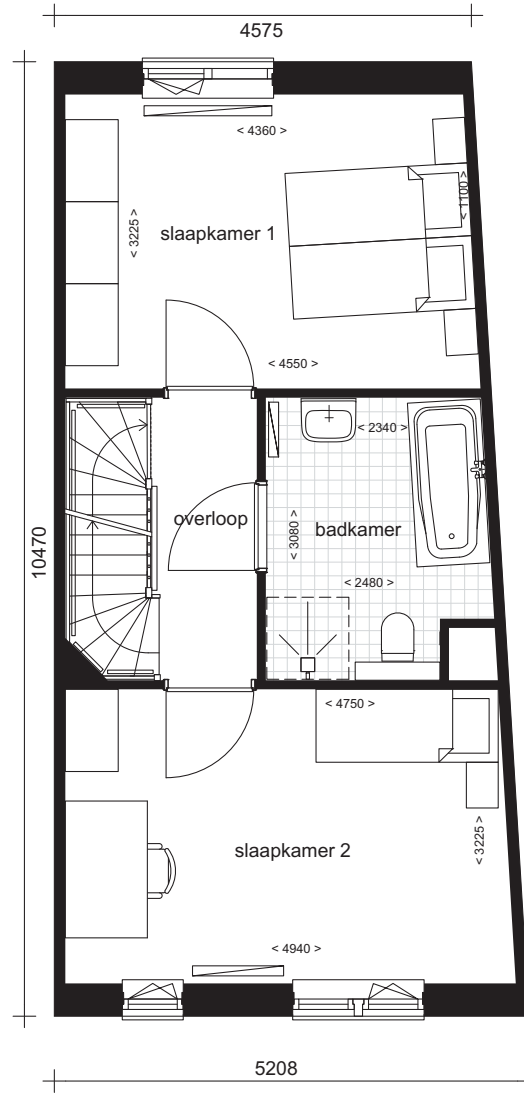
1E VERDIEPING
