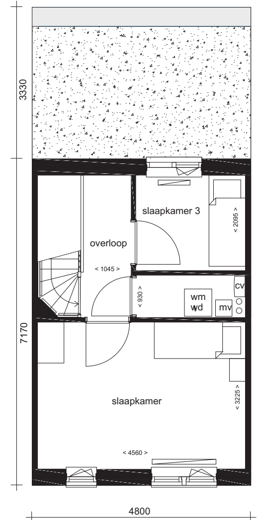
2 E VERDIEPING
